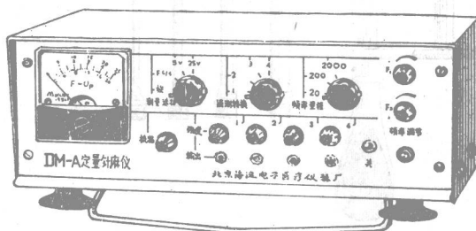
图18 定量针麻仪
