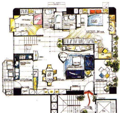
平面设计图
