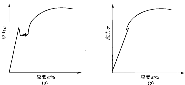
图 1-1 带钢平整前后的应力应变曲线
