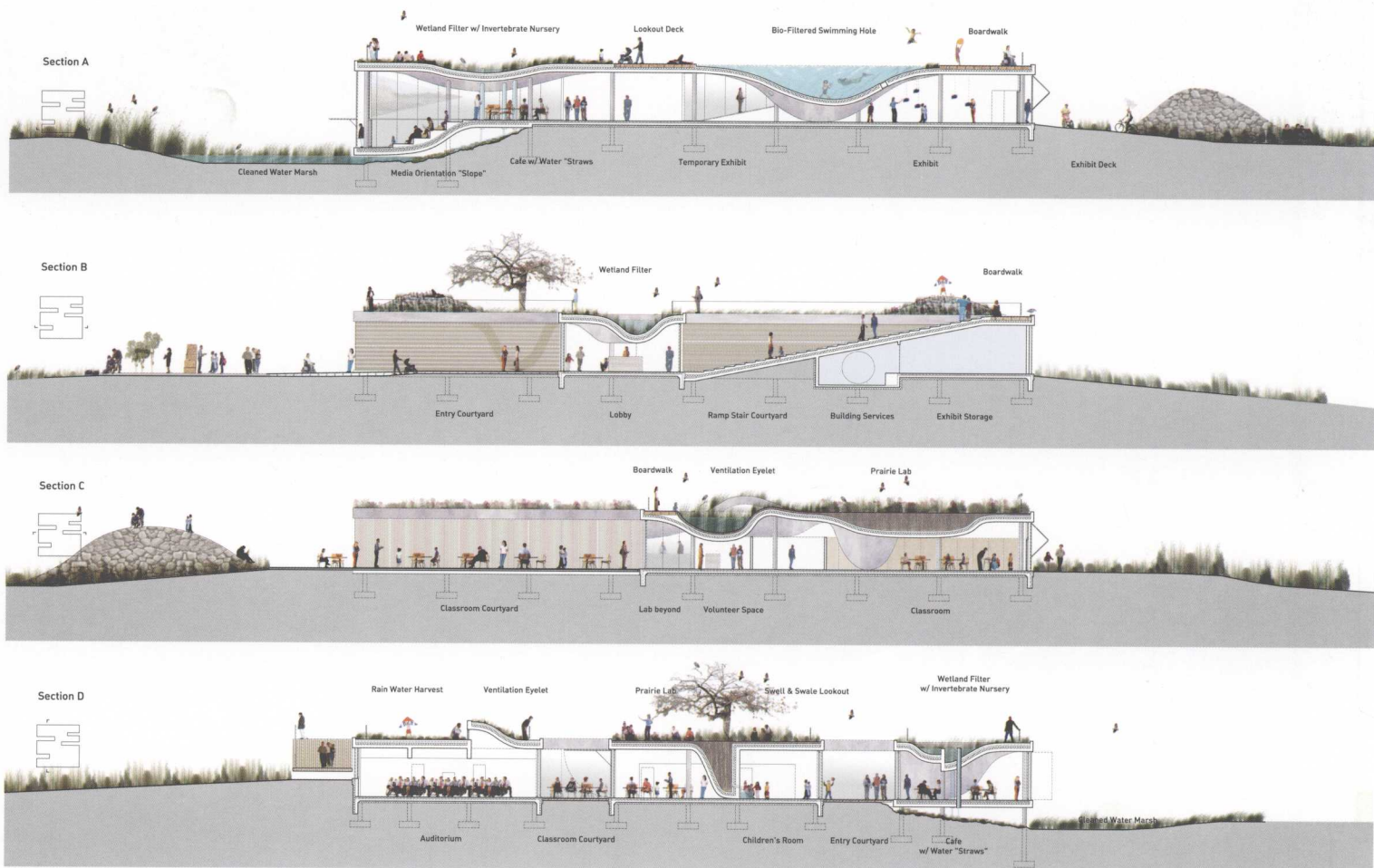
Sections 剖面图
