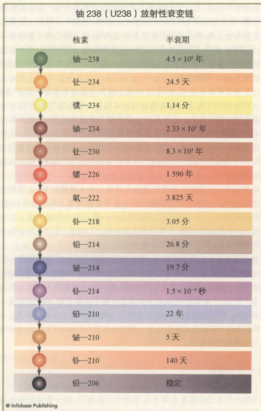
图表 2.1 辐射的种类和不同核素的半衰期
