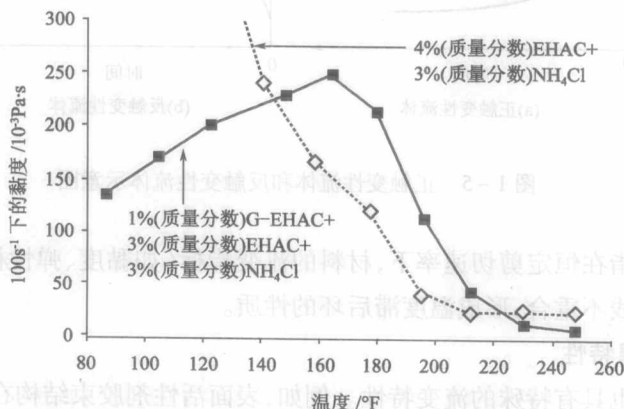
图1-6 G-EHAC与EHAC的黏弹性胶束体系的黏温关系
