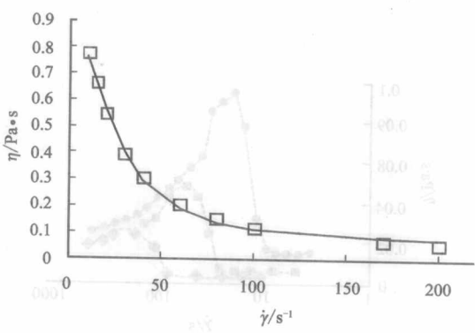
图1-2 黏弹性表面活性剂胶束溶液稳态剪切黏度曲线
