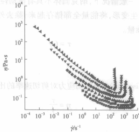
图 1-3 浓矿物颗粒在水中形成的悬浮液的稳态剪切流变性
