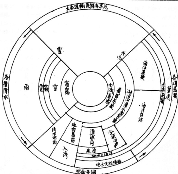
圖 1.2 水循環關係圖
