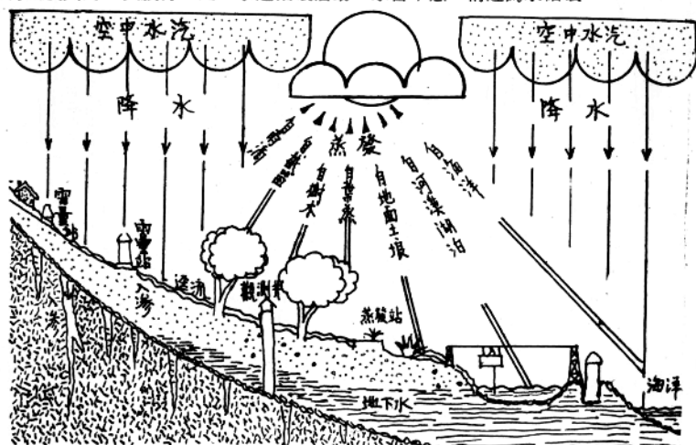
圖 1.1 水循環示意圖
