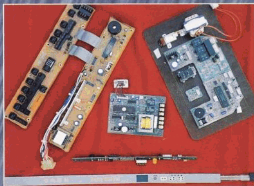
公司生产的高技术、智能型产品——图左上为洗衣机模糊控制器,右上为空调机模糊控制器,中及中下为电冰箱模糊控制器。
