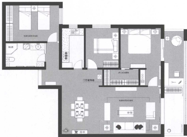
● 平面布置图
