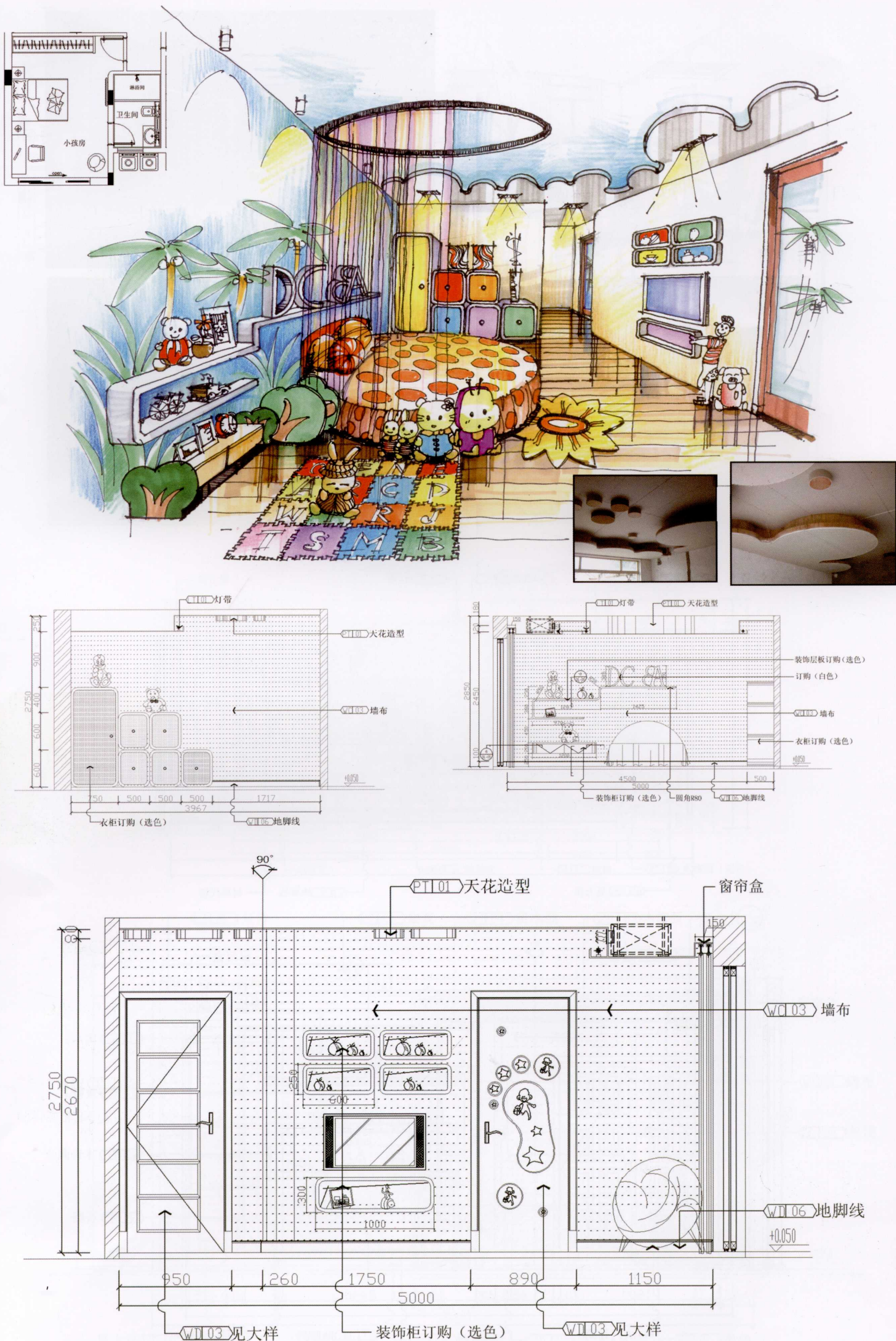
龙先生别墅儿童房设计效果图 (施工图) 文健 赵成余 作
