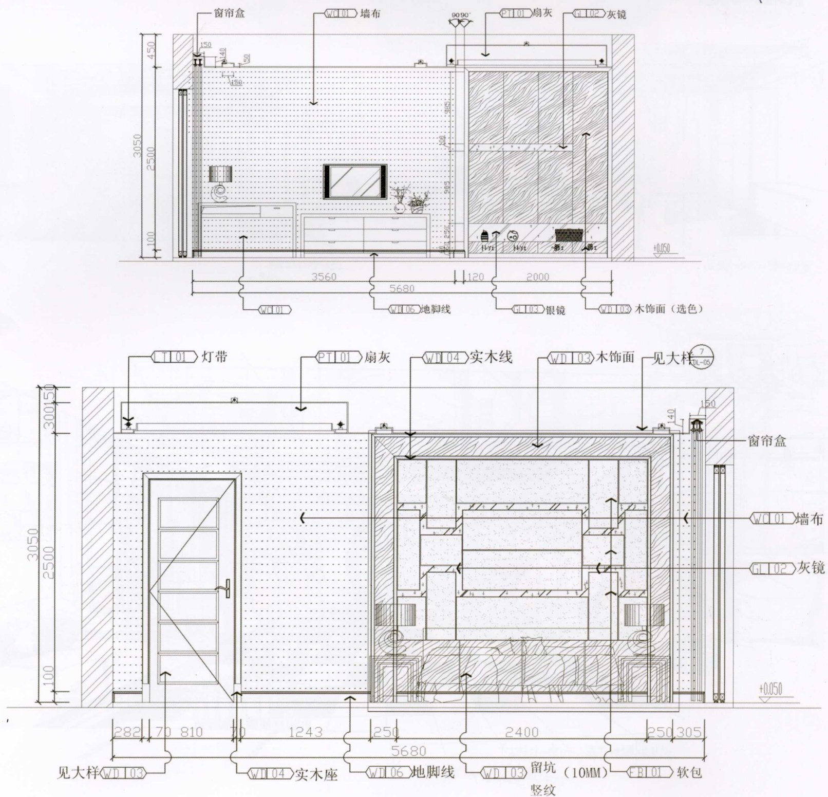
龙先生别墅长辈设计效果图（施工图） 文健 赵成余 作
