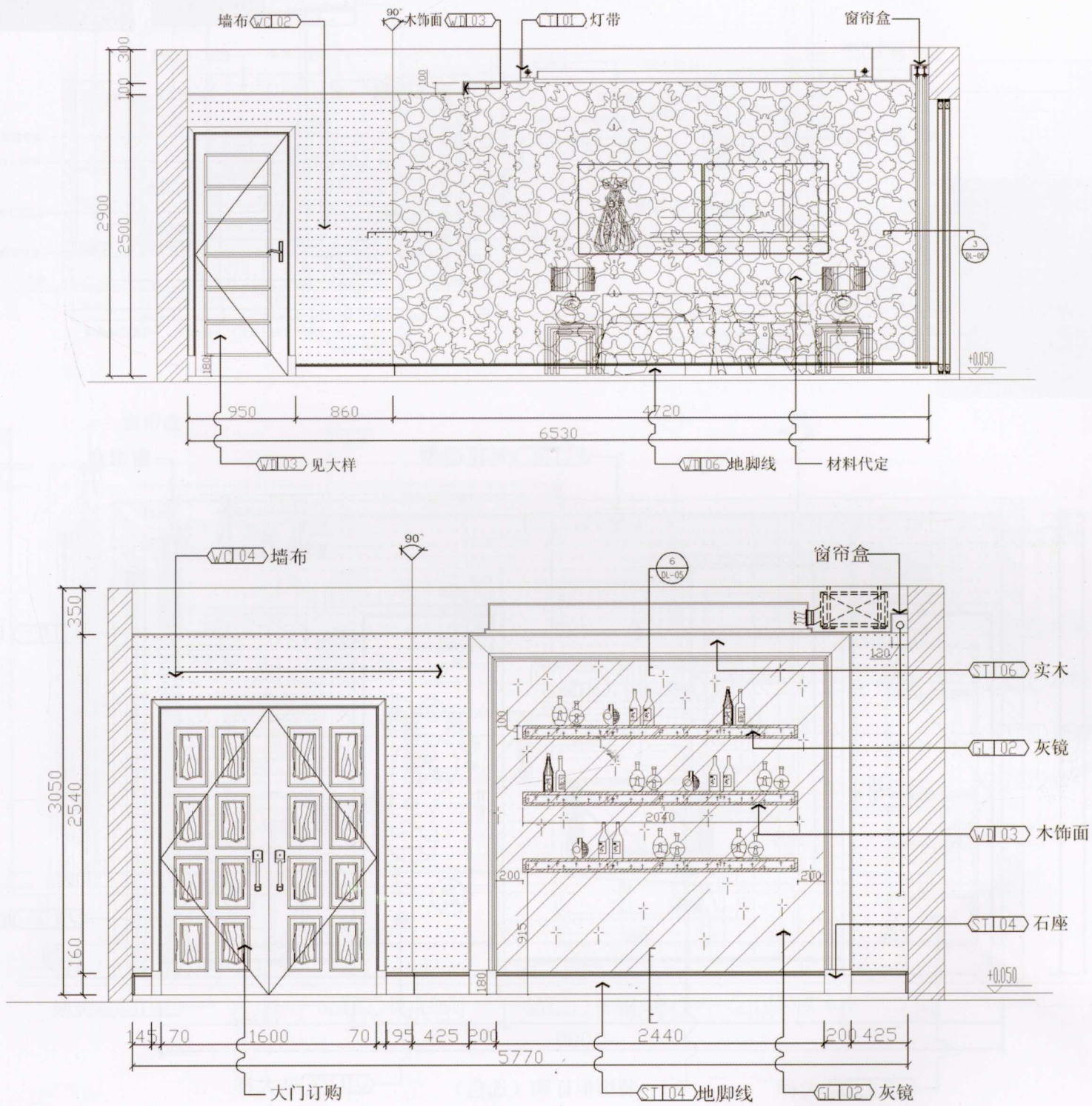
龙先生别墅主卧室、餐厅设计效果图(施工图) 文健 赵成余 作
