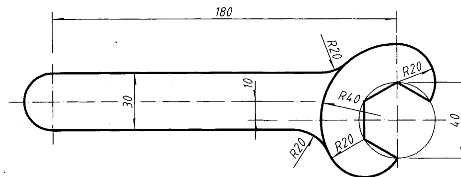
扳手 1:2 (单位mm)
