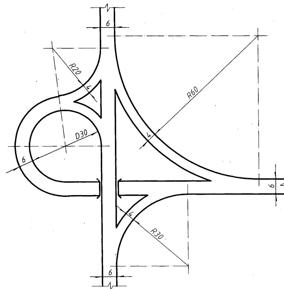
道路交叉口 1:1000 (单位m)
