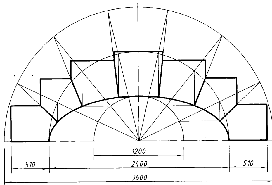
拱门 1:30 (单位mm)
