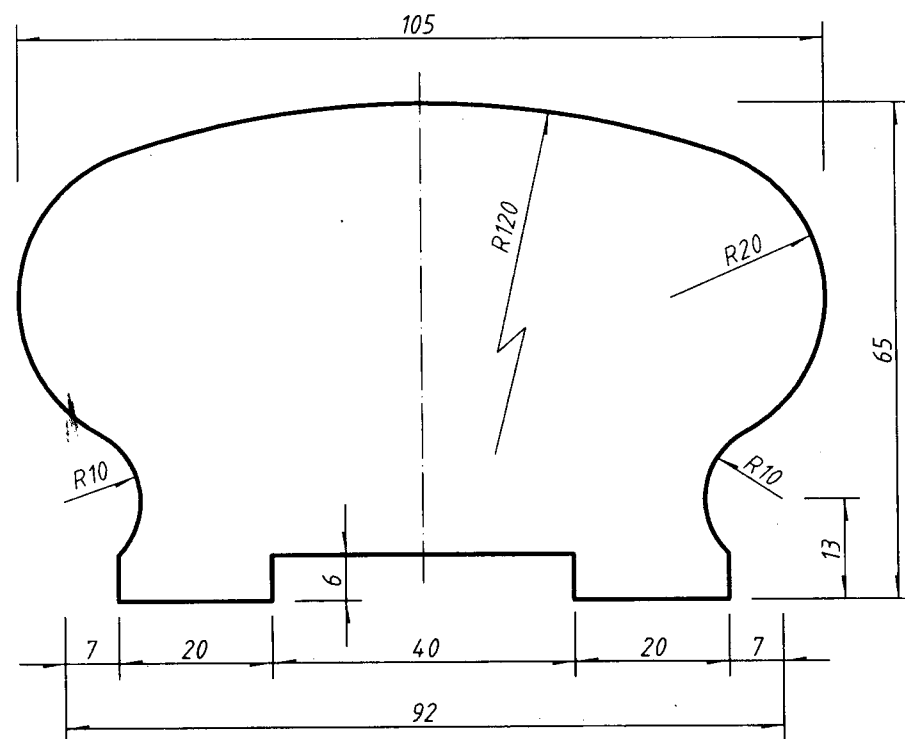
扶手 1:1 (单位mm)
