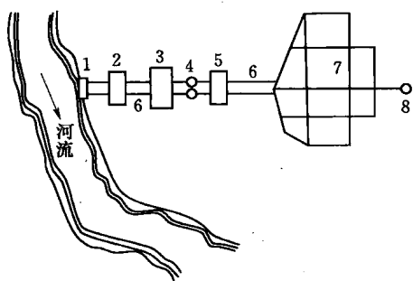
图 1-1 地表水源给水管网系统示意图
