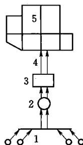
图 1-2 地下水源给水管网系统示意图
