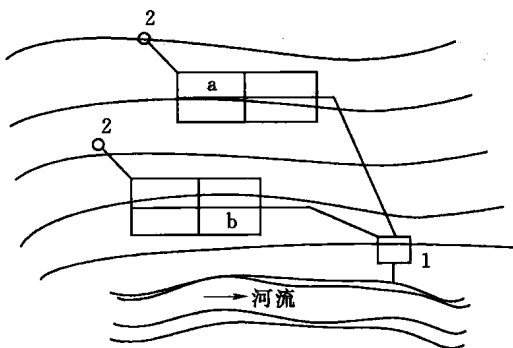
图 1-6 并联分区给水管网系统
