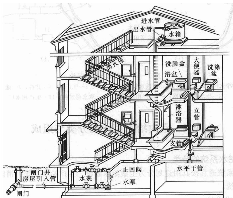
图 1-10 建筑内部给水系统
