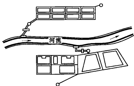
图 1-5 分区给水管网系统
