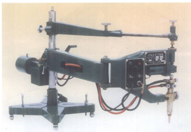
自动仿形气割机
