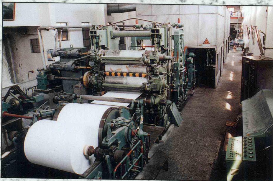
1092双长网多缸造纸机 (新风铜网造纸厂)
