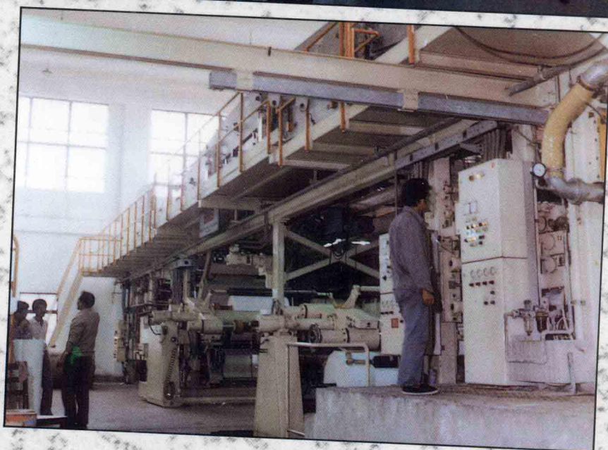
生产无碳复写纸涂布机 (感光复印纸厂)
