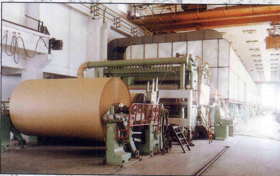
年产5万吨牛皮箱板纸机(宏文造纸厂)
