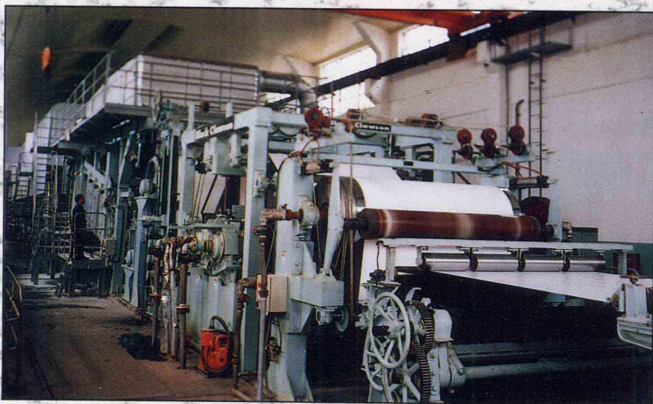
涂布白板纸机(中国版纸厂)
