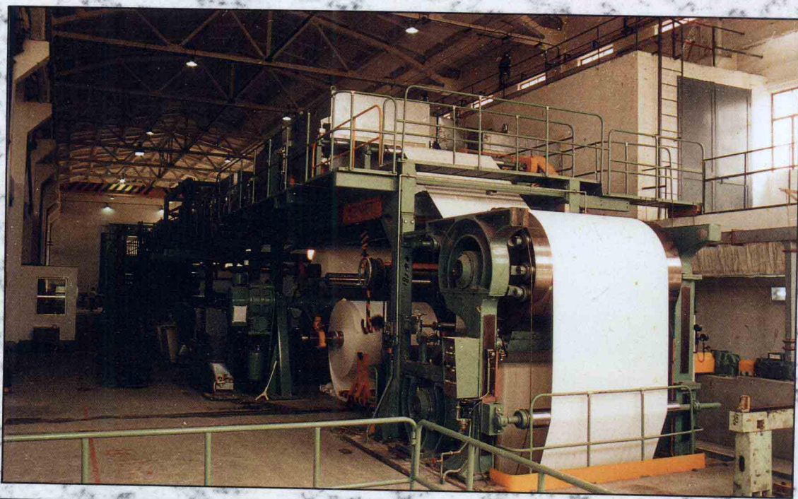
1800毫米四刮刀涂布机
