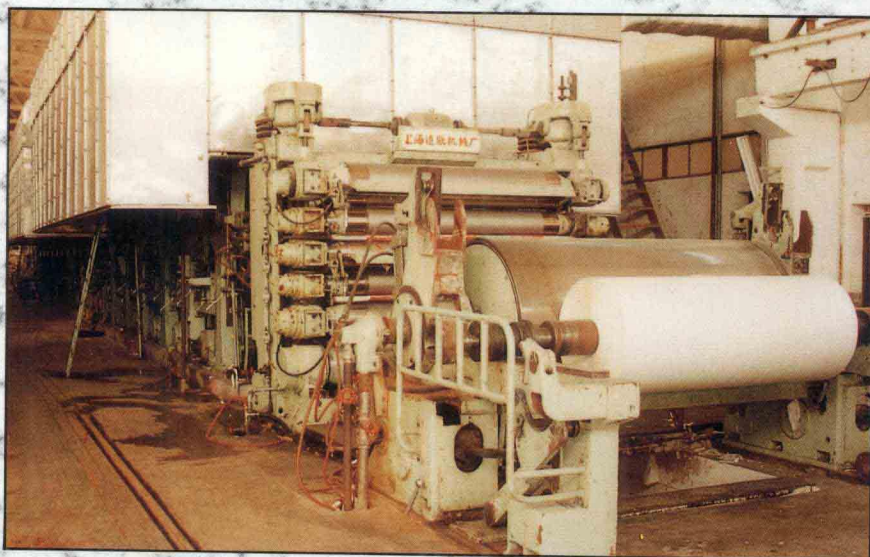
1092双长网多缸造纸机 (新风铜网造纸厂)
