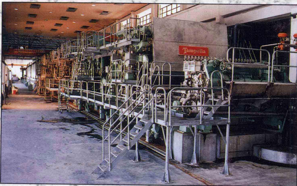
高级折叠涂布白板纸机(星火制浆造纸厂)
