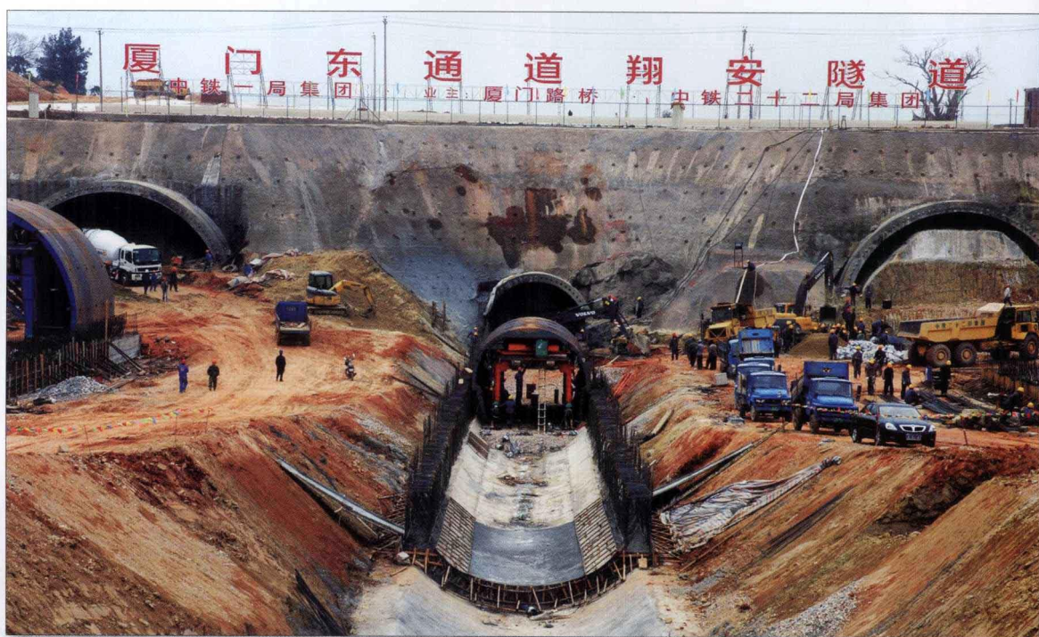
4月30日，祖国大陆第一条大断面海底隧道——翔安隧道正式动工。图为施工现场。（陈立新 摄）
