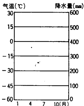
气温年变化和降水量月份分配图
