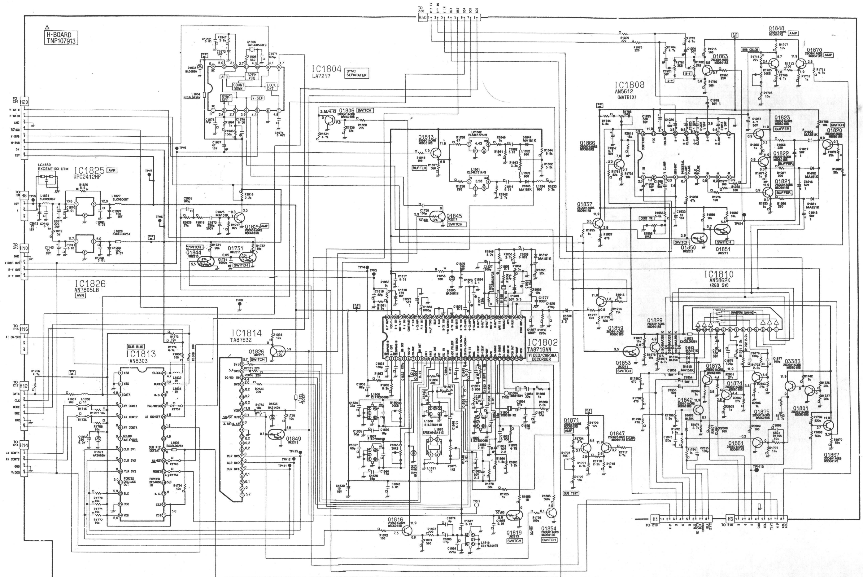
松下TC-33V30H 画中画处理电路(数字伴音电路参见TC-29V2H,主机芯电路同松下TC-29V30R)
