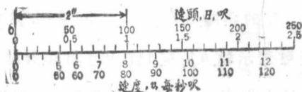
圖 3. 速度變換成速頭
