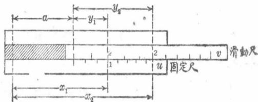
圖 5. 一滑動尺和一固定尺合成的算尺
