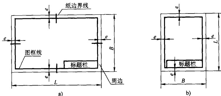
图 1-1 不留装订边的图纸格式
