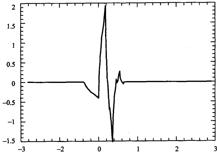
图 5 高频 Daubechies 小波
