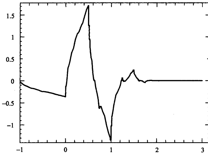
图4 Daubechies 小波
