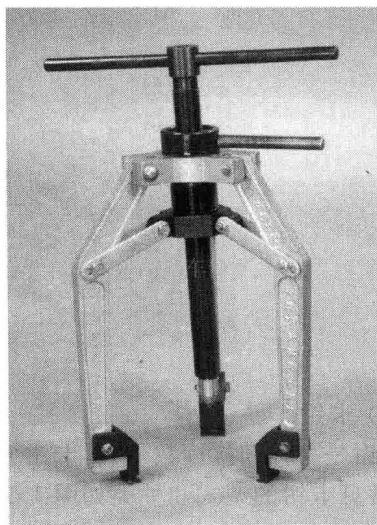
图 1.13 变速箱轴承拉器
