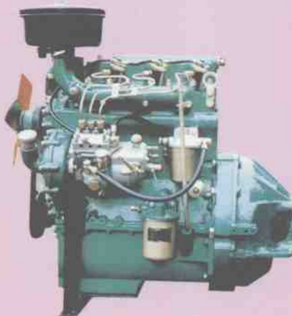
390型柴油机
