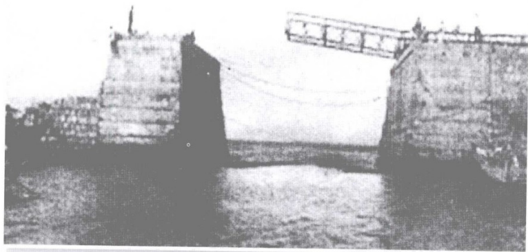
在两个巨大的沉箱上，用条石砌起桥墩。桥台高耸，贝雷式桥梁缓缓推进。
