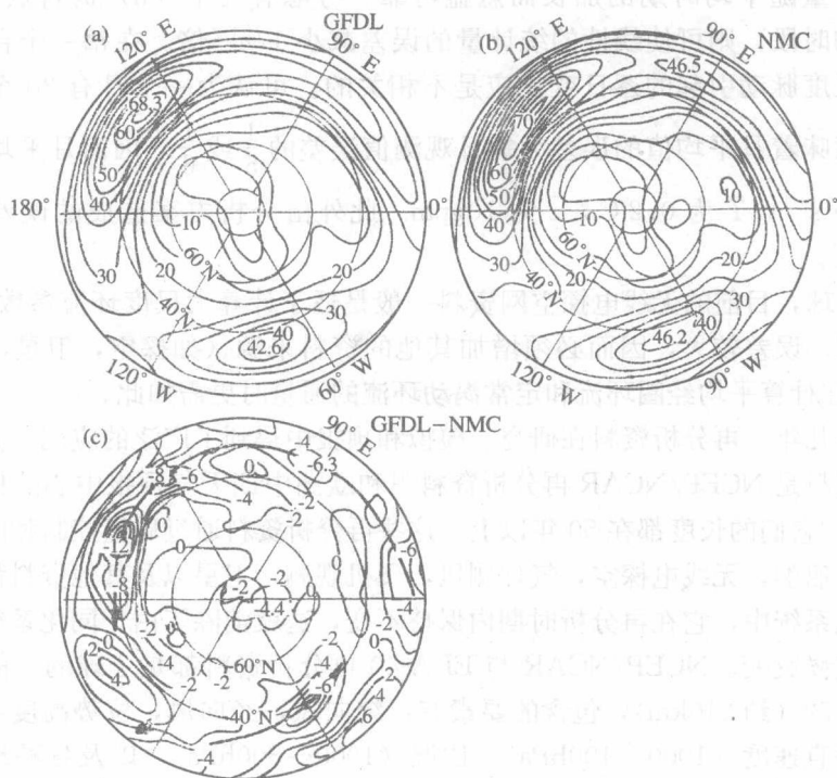
图 1.2 9 个冬季 (1963~1973) 200hPa 纬向风分布 [6]
