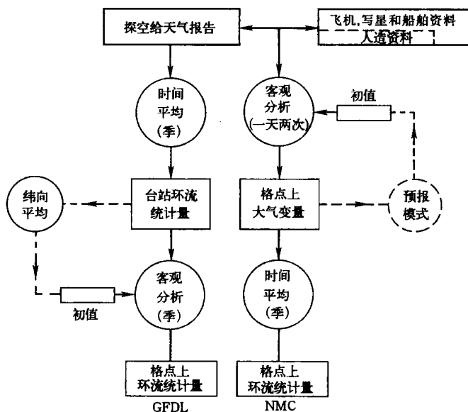
图 1.1 用于大气环流研究的两种资料处理方法的比较 [4]
