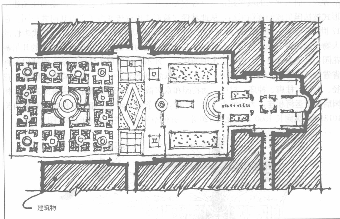
图 1-1 意大利白齐诺雅的朗俄托别墅平面
