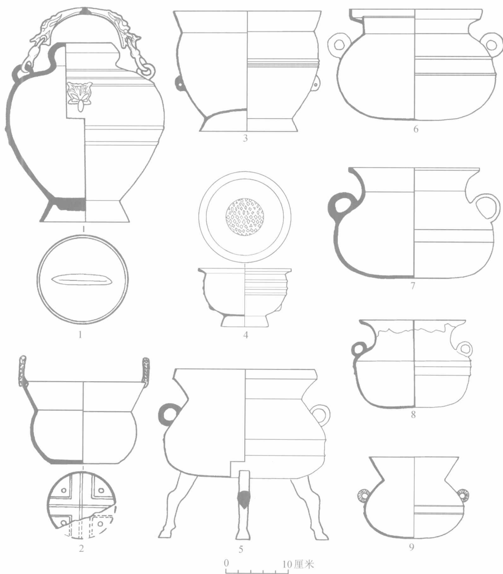
图五八一 汉式墓出土的铜壶、釜、甗、鼎及釜
