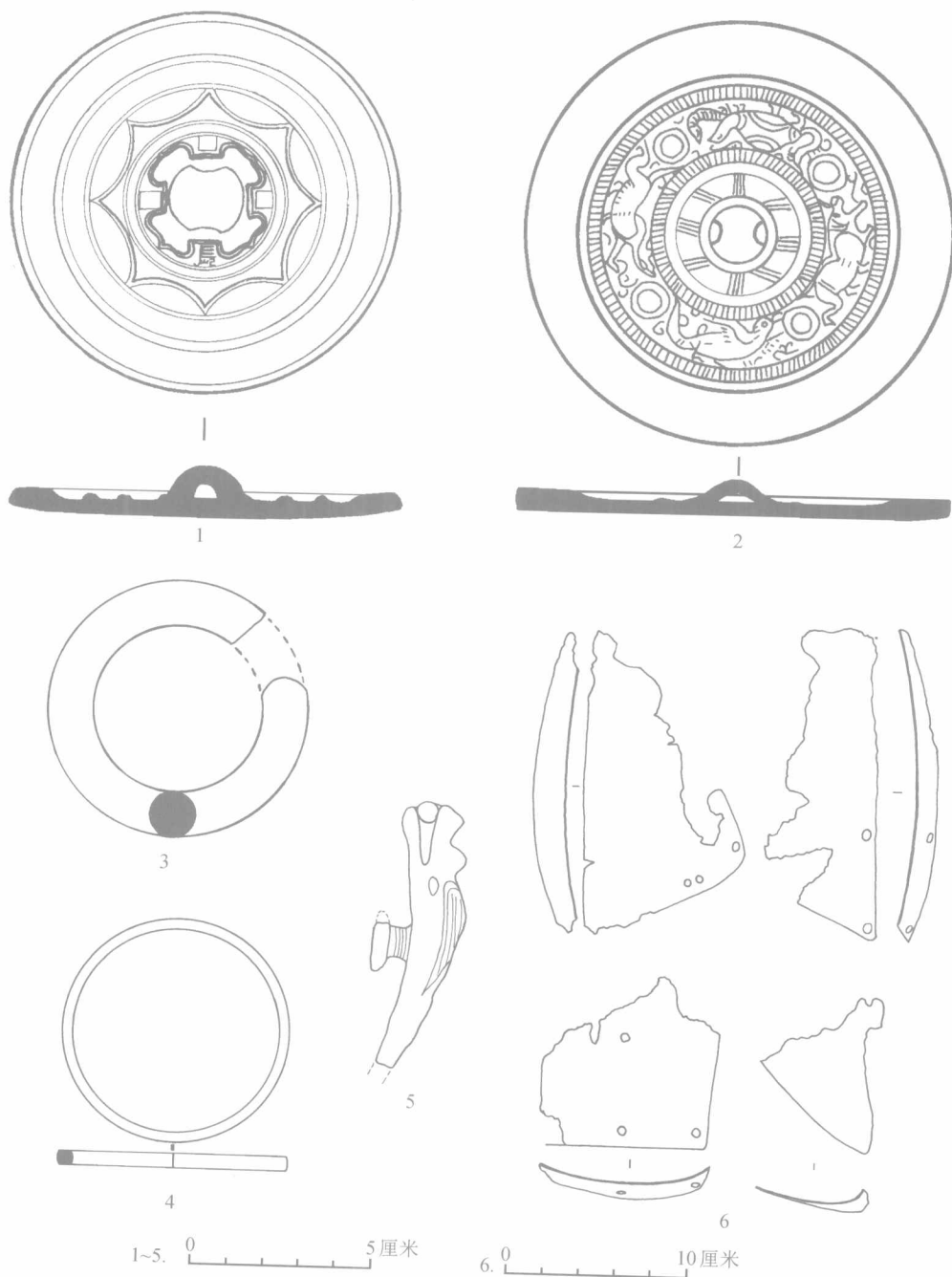
图五八四 汉式墓出土的铜镜、钁、带钩及臂甲
