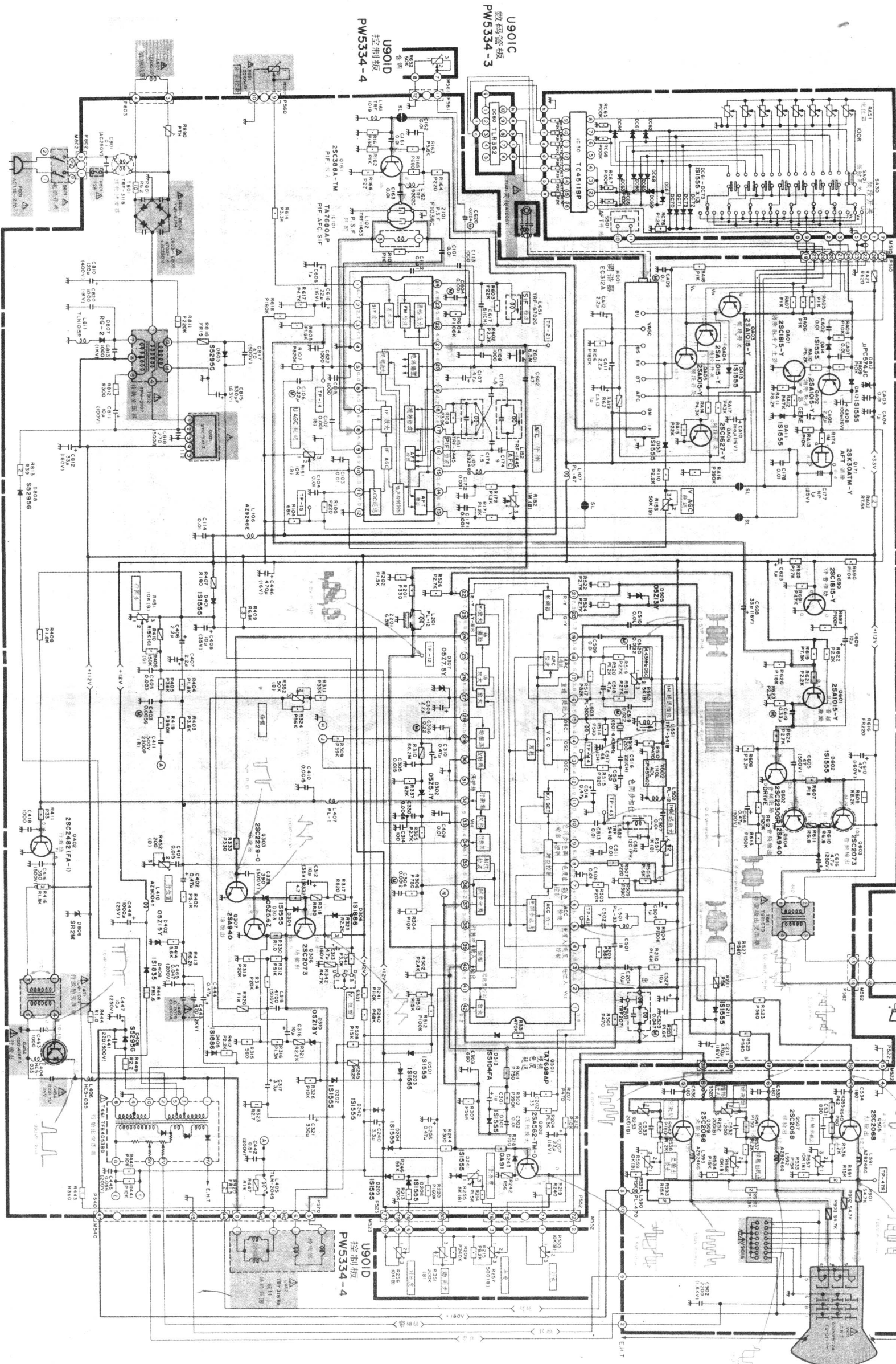
电路图
