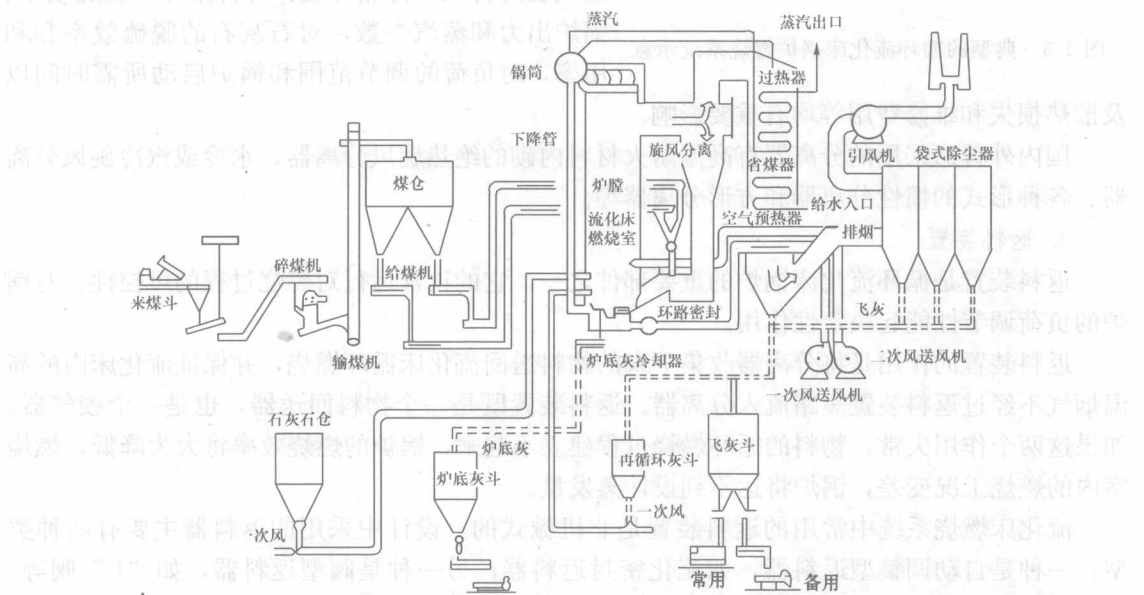
图 1-2 循环流化床锅炉的工作过程
