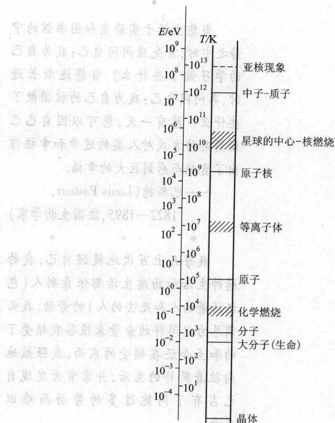
图1 量子阶梯
