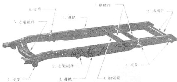
圖2-7 典型的大貨車車架
