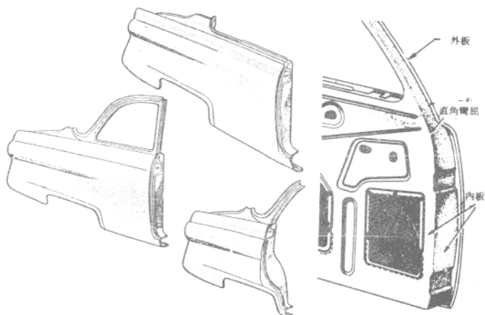
圖3—3 直角彎屈的內門板
