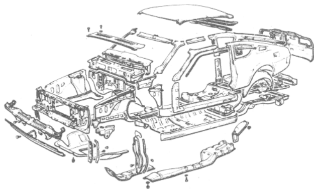
圖 1—3 現代汽車車身的構成件
