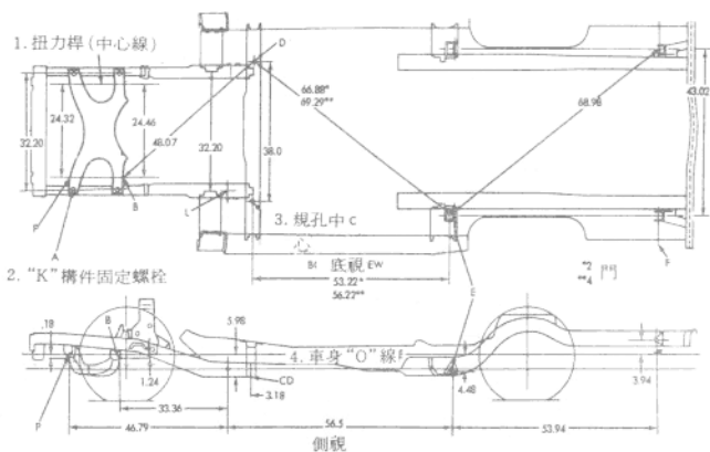
圖2-6 短柱架車架
