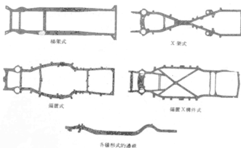
圖2-1 車架的各種型式
