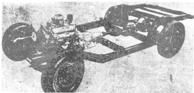
圖2-3 準備裝上車身的底盤架
