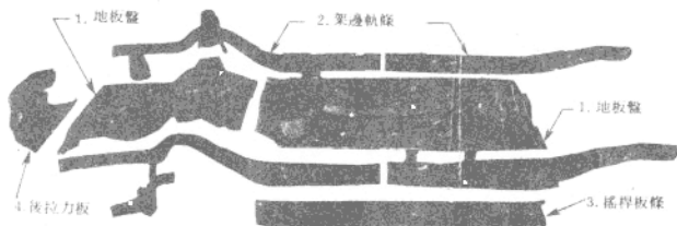
圖2-5 車架與下體的整體結構
