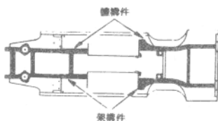
圖2-4 體與架整體結構頂視圖
