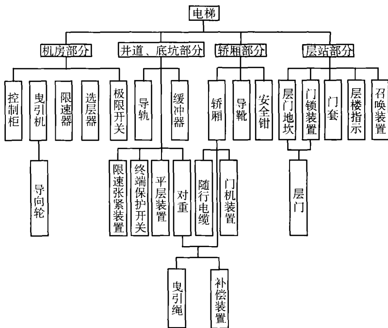
图 1.1.5 电梯各装置（部件）放置位置示意
