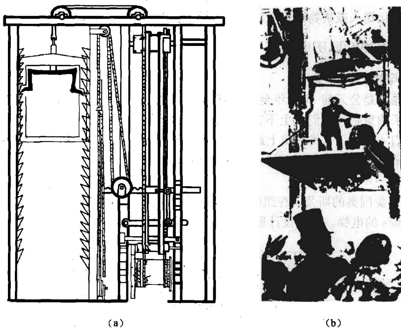
图 1-1.2 美国人奥的斯表演他设计成功的安全装置
