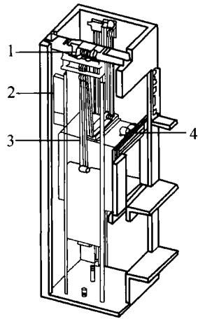
图 1.1.7 无机房电梯的构造
