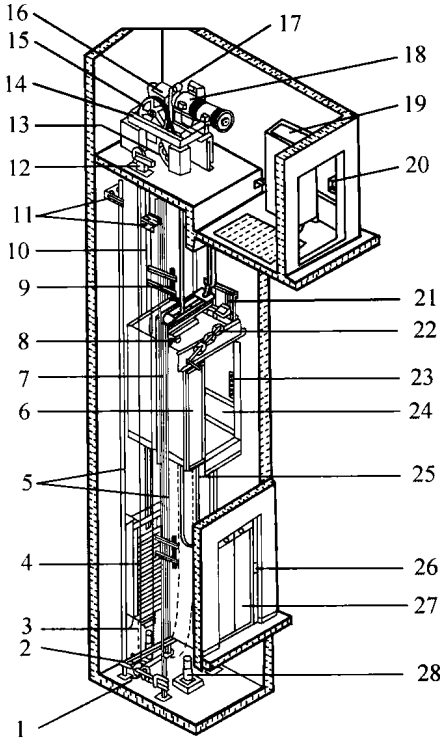
图 1.1.6 电梯的基本构造
