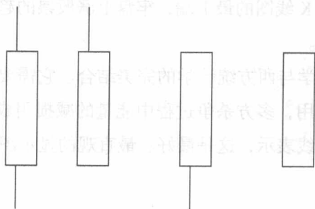
图 1-2 大阳线图
