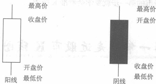
图 1-1 K 线图
