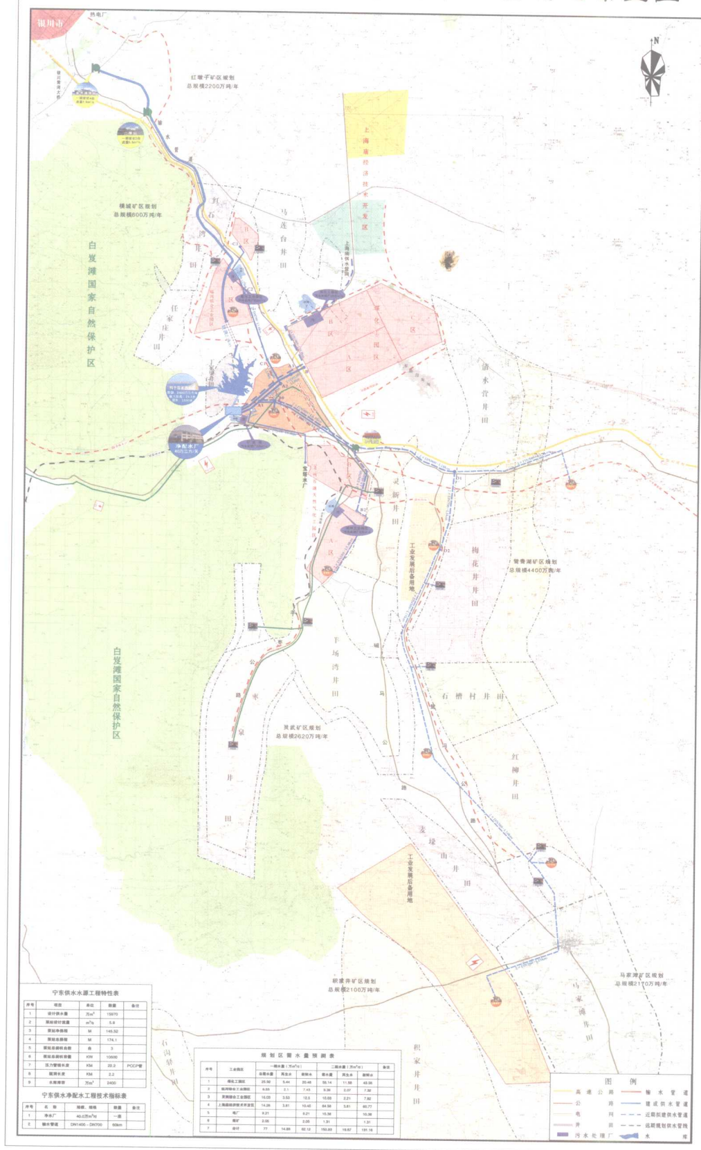
宁东能源化工基地供水工程规划布置图
