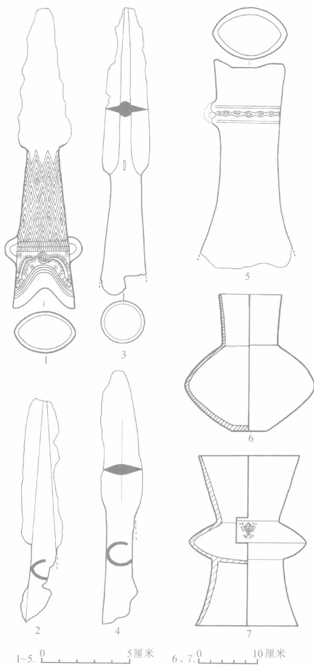
图二八七 M6 随葬器物
