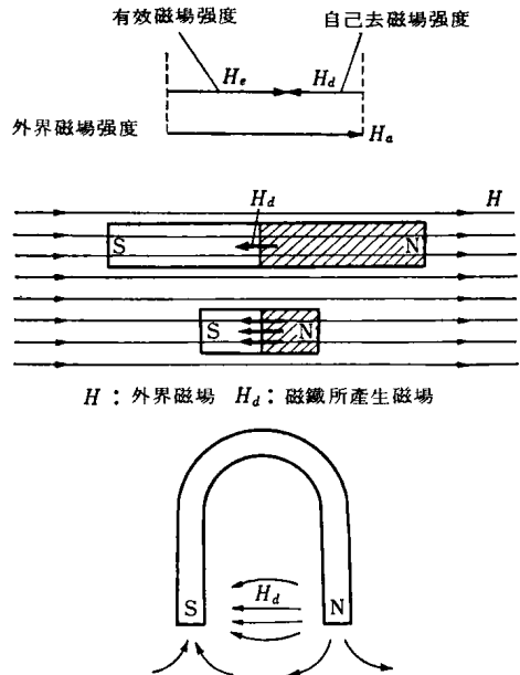
圖 1.1 永久磁鐵與去磁場與形狀之關係 去磁場為負作用，磁鐵之磁化強度減弱， ( 仍朝着正方向 )
