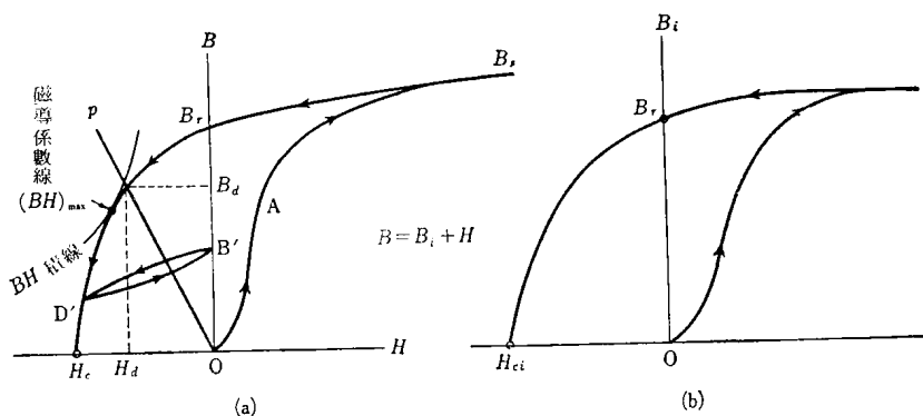
圖1.2 磁化曲線（ OAB_s ）與去磁曲線（ B_rD'H_c ）
