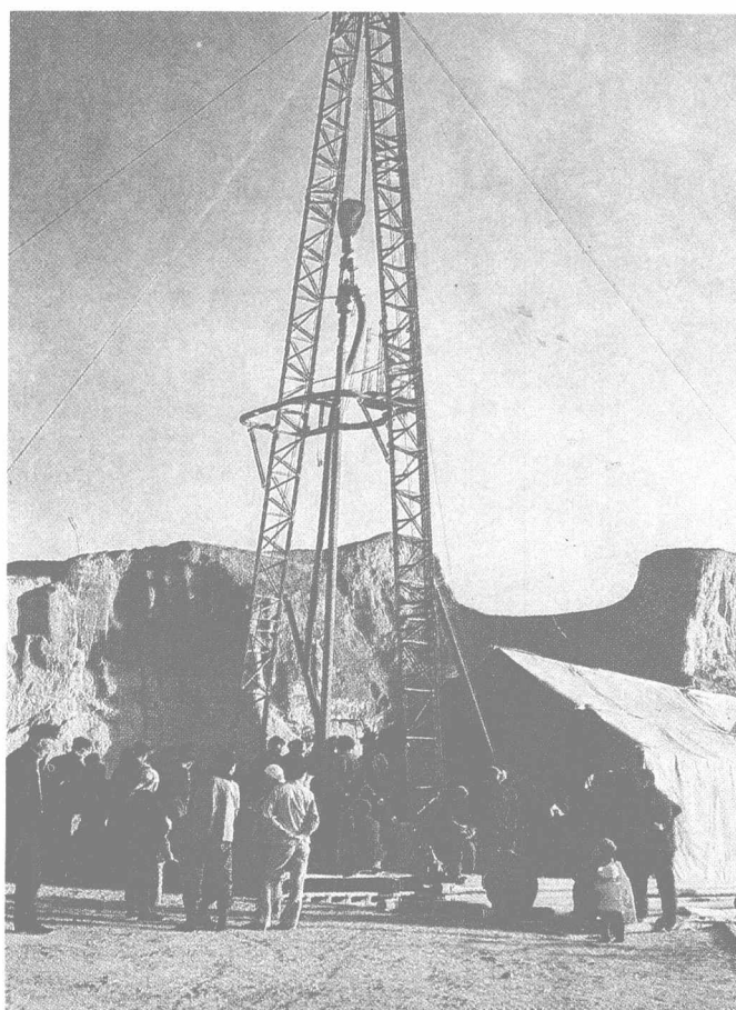
机械打井
