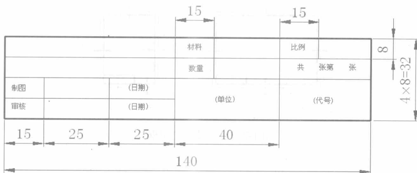
(a) 零件图标题栏
