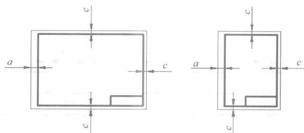
图 1-3 留装订边图框
