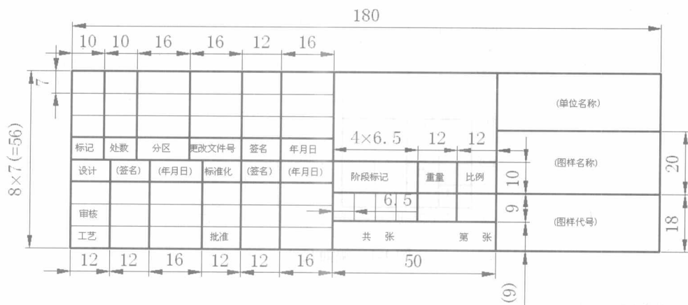
图 1-4 标题栏
