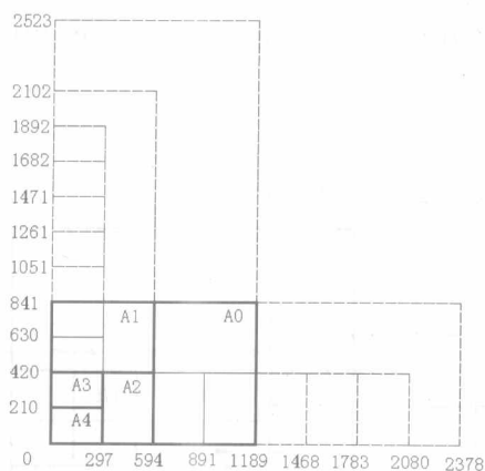
图 1-1 幅面尺寸
