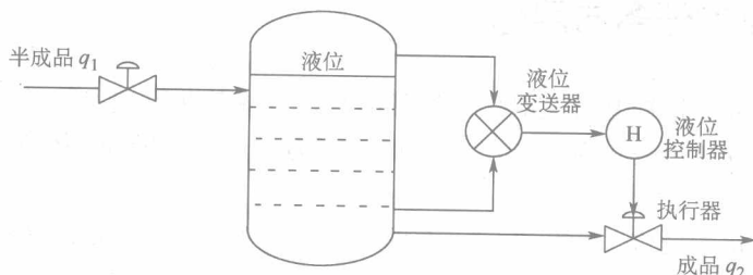
图 1-1 水槽液位控制系统
