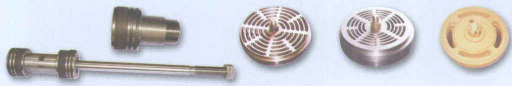
连体式活塞气阀
