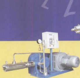
◇ DYB系列低温液体泵
