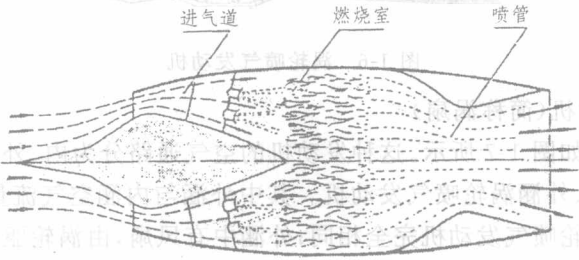
图 1-4 冲压式喷气发动机
