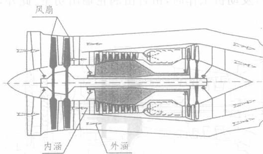
图 1-7 涡轮风扇发动机
