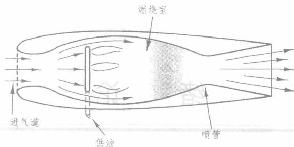
图 0-2 罗兰型喷气发动机
