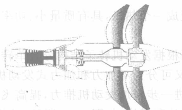
图 1-8 桨扇发动机
