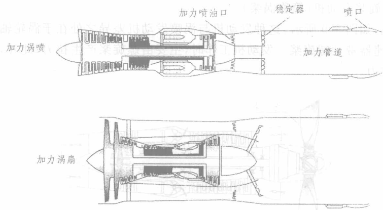
图 1-11 加力燃烧
