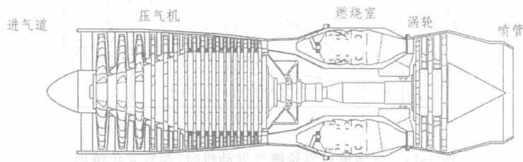
图 1-13 单轴轴流式涡轮喷气发动机
