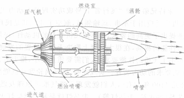
图 0-3 惠特利型的一种涡轮喷气发动机
