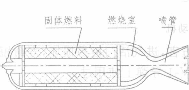
图 1-2 固体燃料火箭发动机
