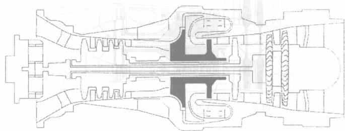
图 1-10 涡轮轴发动机
