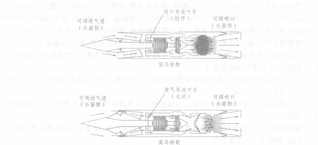
图 1-12 涡喷—冲压组合发动机
