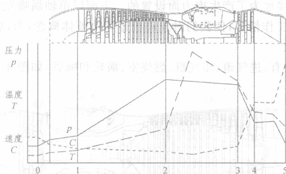
图 1-14 气体流过涡轮喷气发动机时,参数变化情形
