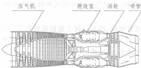
图 1-6 涡轮喷气发动机
