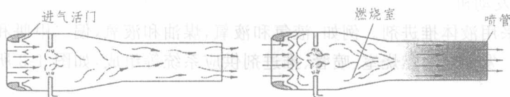
图 1-5 脉动喷气发动机
