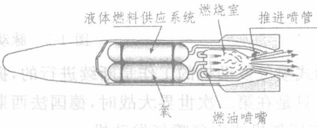
图 1-3 液体燃料火箭发动机
