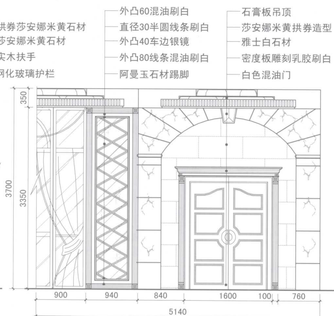
B 3 客厅立面图 Elevation(Living Room)
