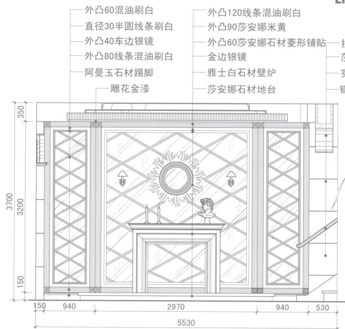
A 3 客厅立面图 Elevation(Living Room)
