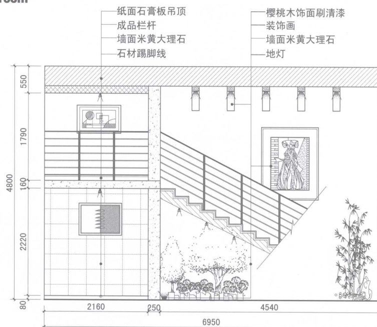
客厅长立面 Elevation(Living Room)
