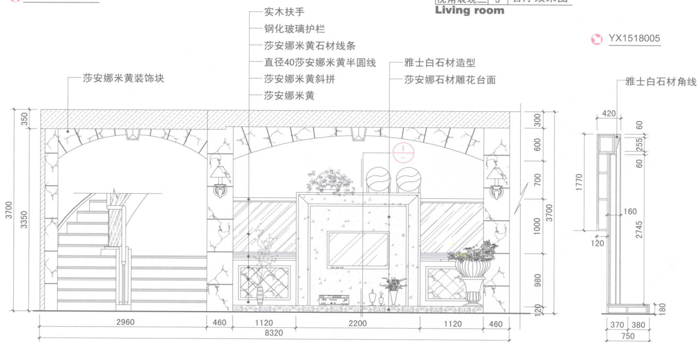
C 3 客厅立面图 Elevation(Living Room)
