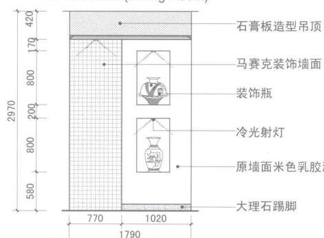
客厅立面图 Elevation(Living Room)
