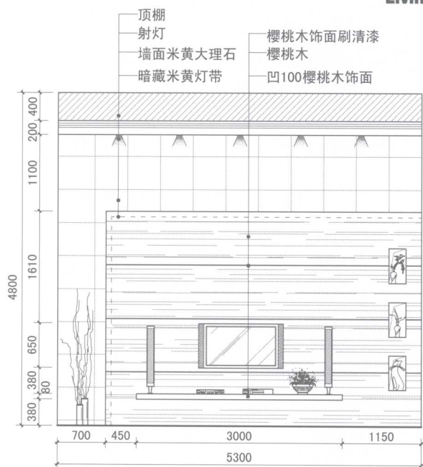
客厅长立面 Elevation(Living Room)
