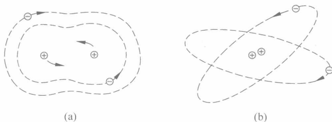
图 12.2 氢分子(a)与氦原子(b)结构示意图
