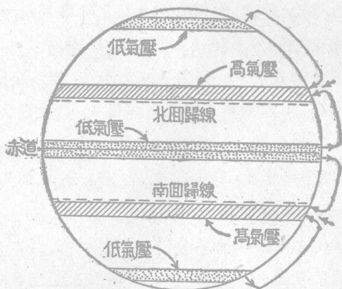
地球上氣壓帶的分佈和高空的氣流
