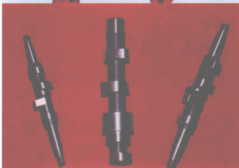
凸 轮 轴
