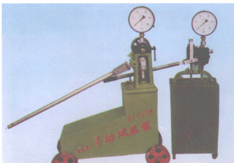
试 压 泵
