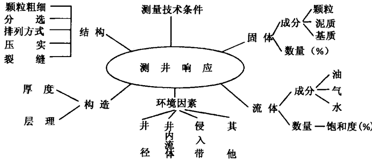
图 1-4 影响测井响应的各种因素
