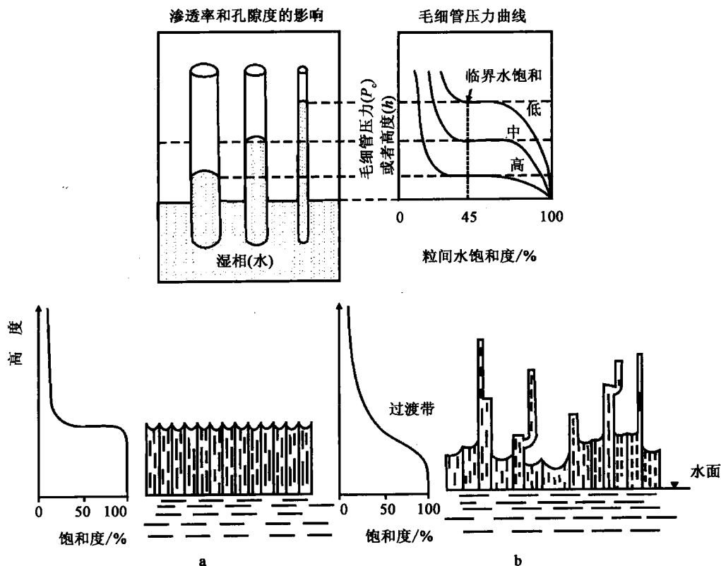
图 1-3 毛细管压力曲线和孔隙结构关系
