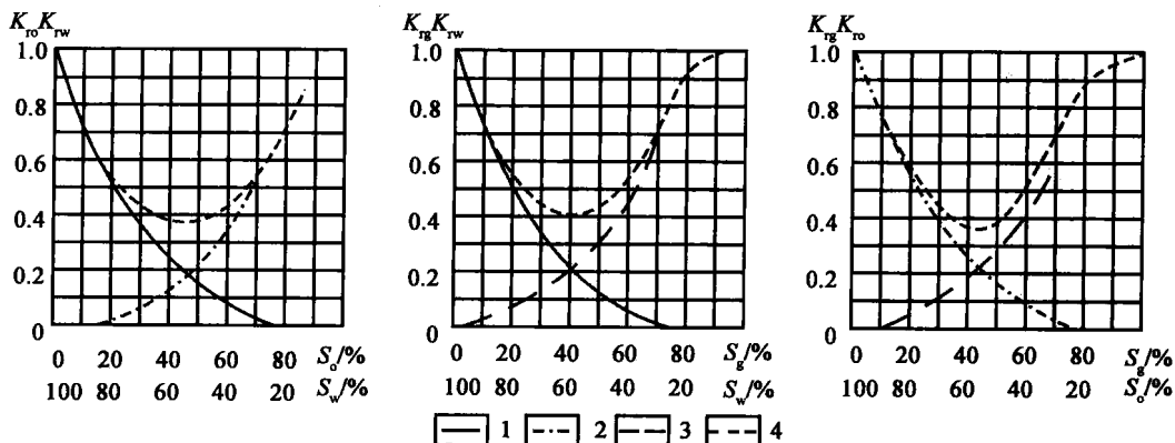
图 1-1 相对渗透率与饱和度的关系
