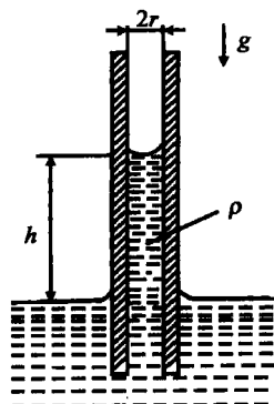
图 1-2 毛细管中水面增高
