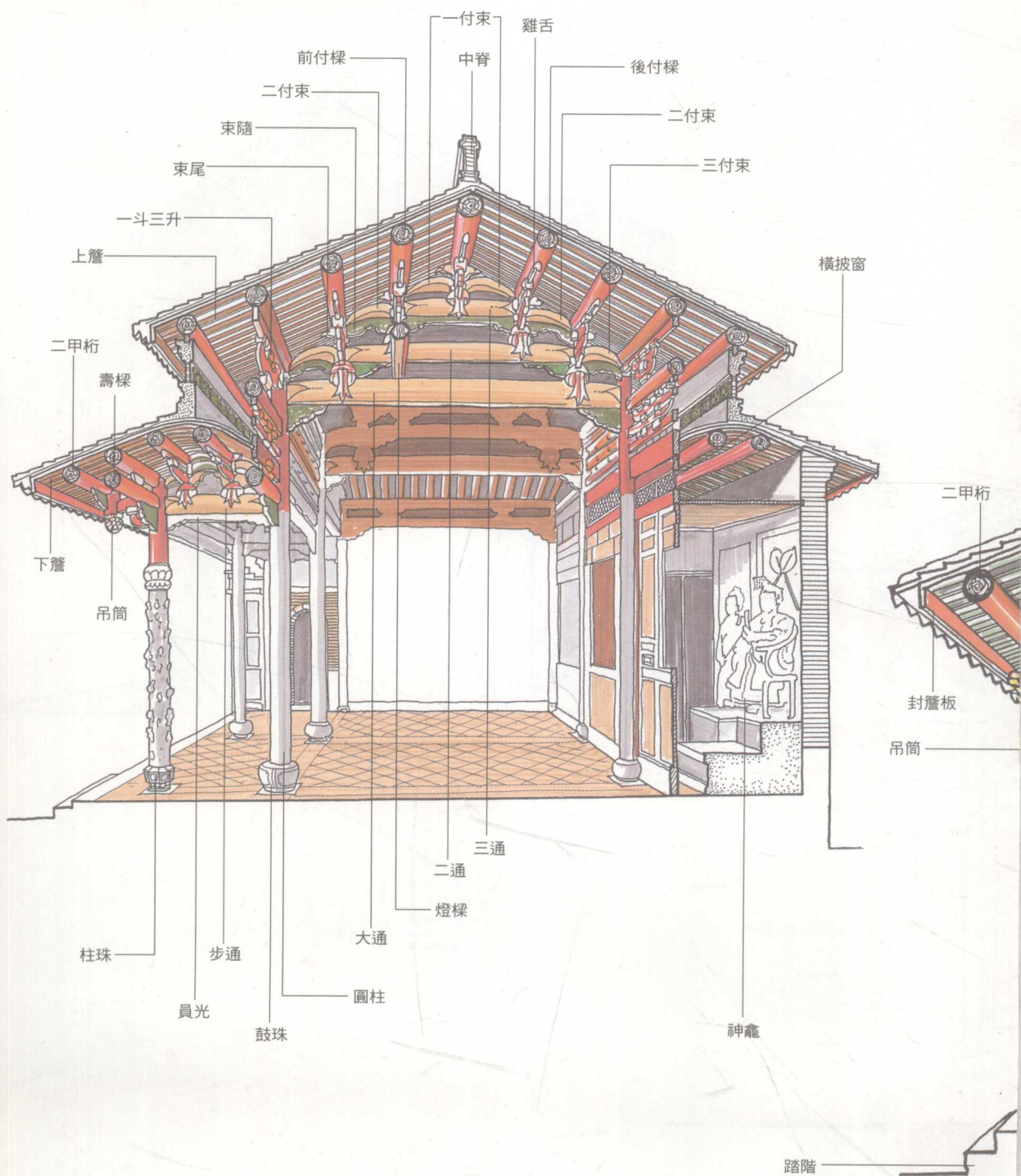
艋舺龍山寺後殿構造分解圖【彩圖八】
