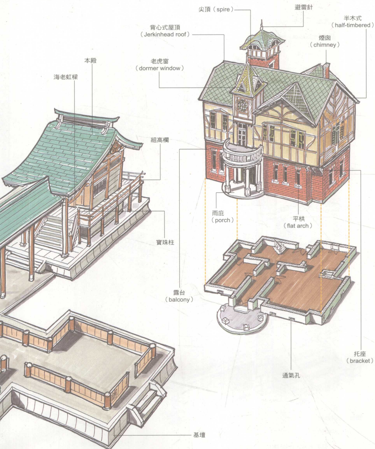
台北圓山別莊構造分解圖 [彩圖十三]
