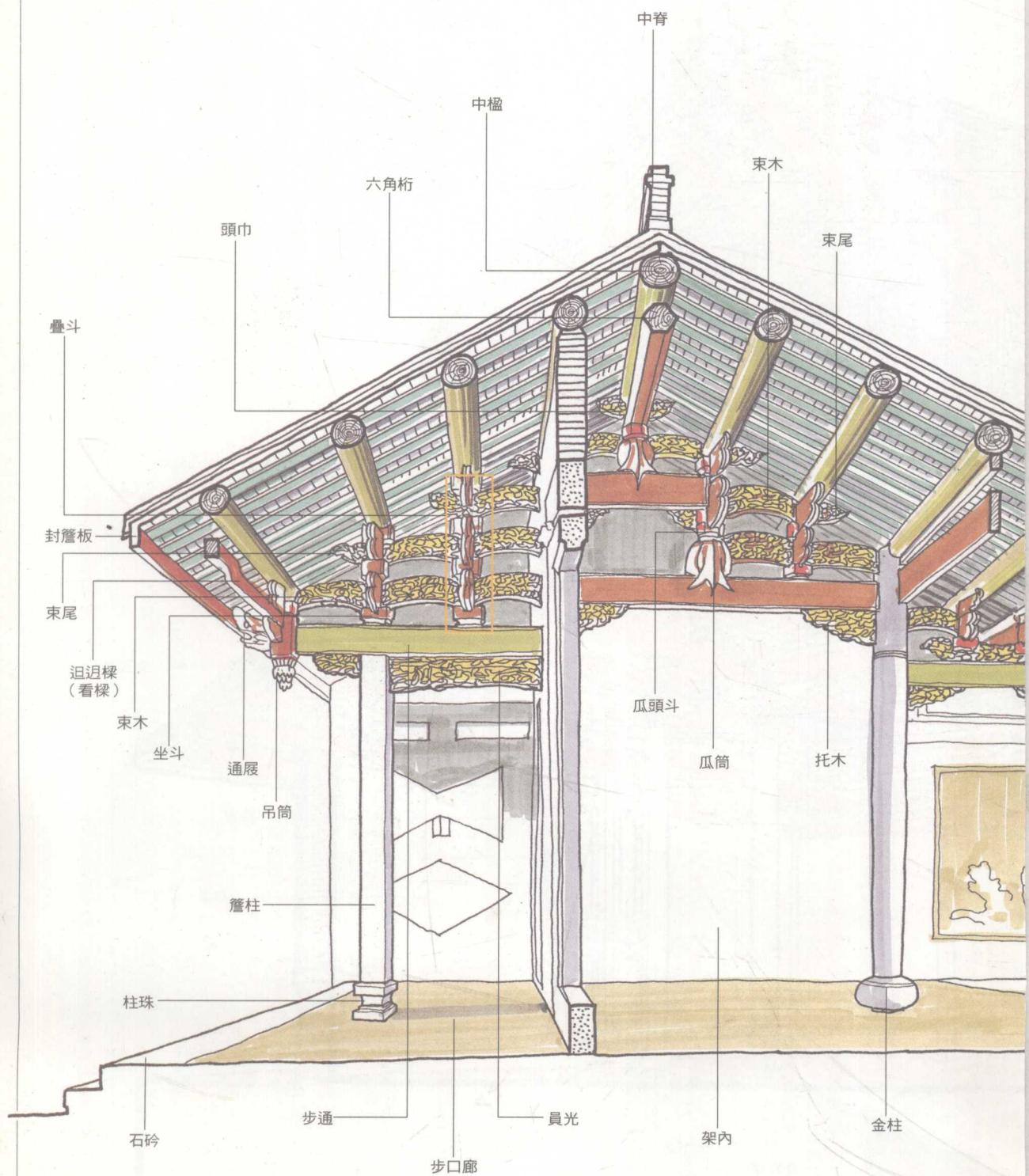
台南三山國王廟前殿構造分解圖〔彩圖六〕
