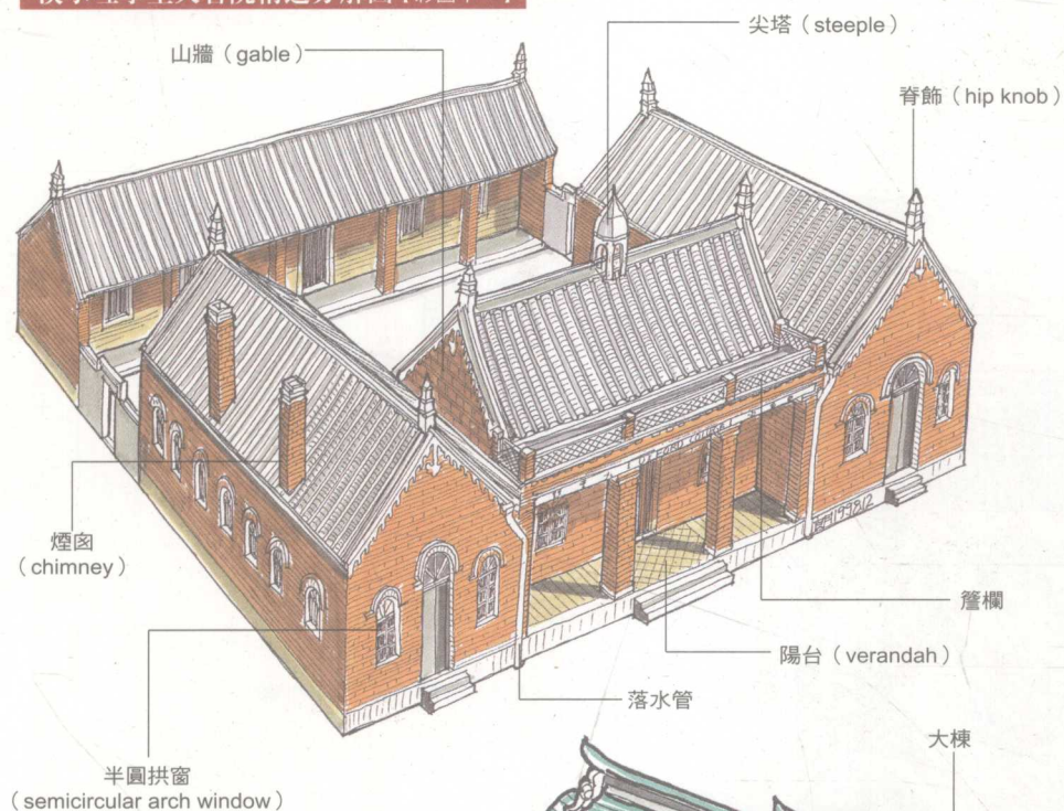
淡水理學堂大書院構造分解圖【彩圖十一】
