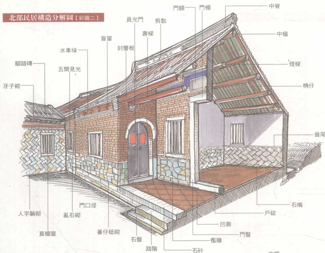
澎湖民居構造分解圖 (彩圖三)
