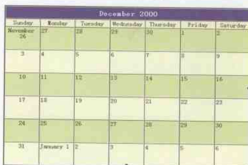
图 14-21 (日历插件)
