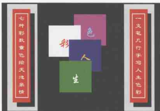
图 10-18 (图层的应用)
