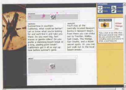
图 15-62 (使用模板)
