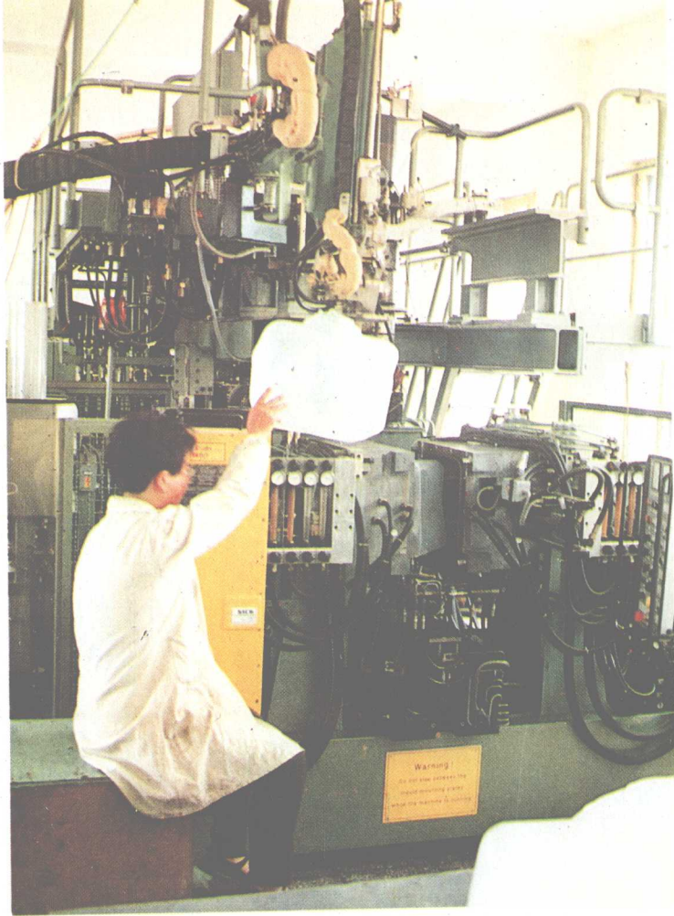
22 长春工贸合营塑料制品厂生产线
