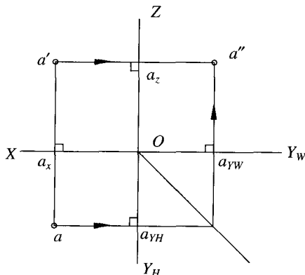
(b) 作图
