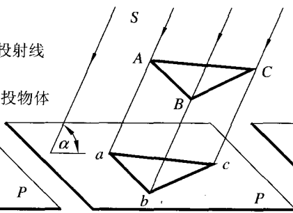
图 1-2 斜投影
