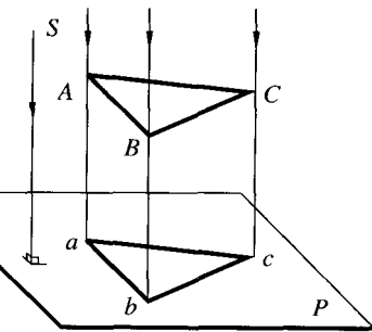
图 1-3 正投影
