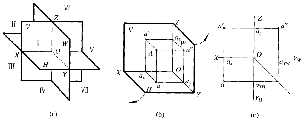
图 2-5 三面投影体系及其点的投影
