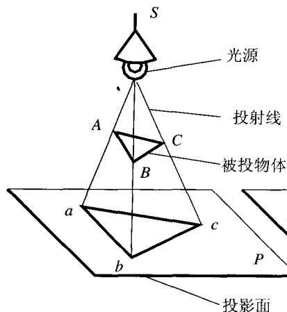
图 1-1 中心投影
