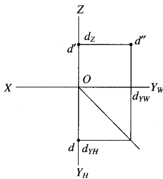
(b) 图解
