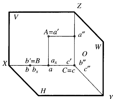
(a) 直观图
