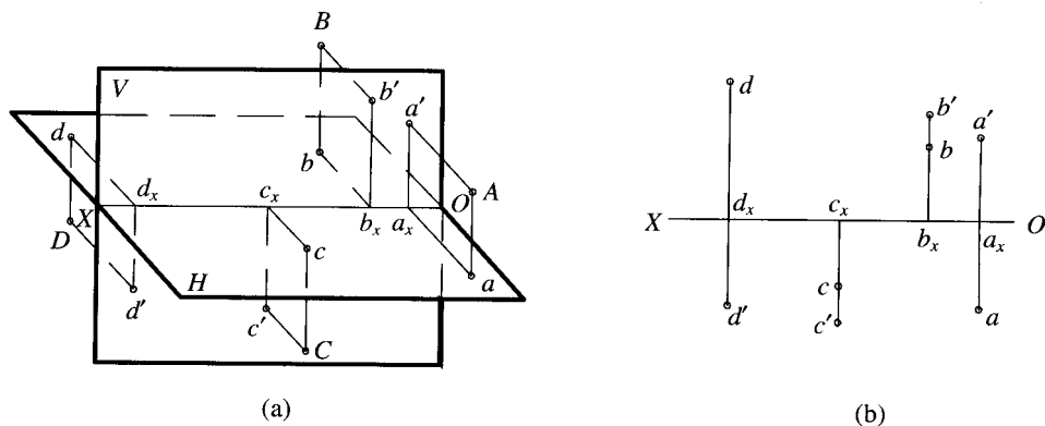
图 2-4 各分角内点的投影
