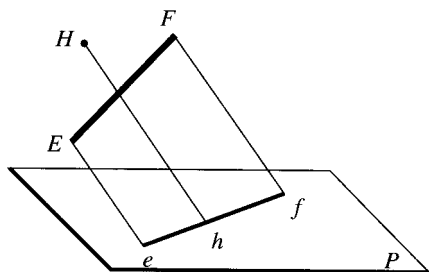
图 1-7 H \notin EF
