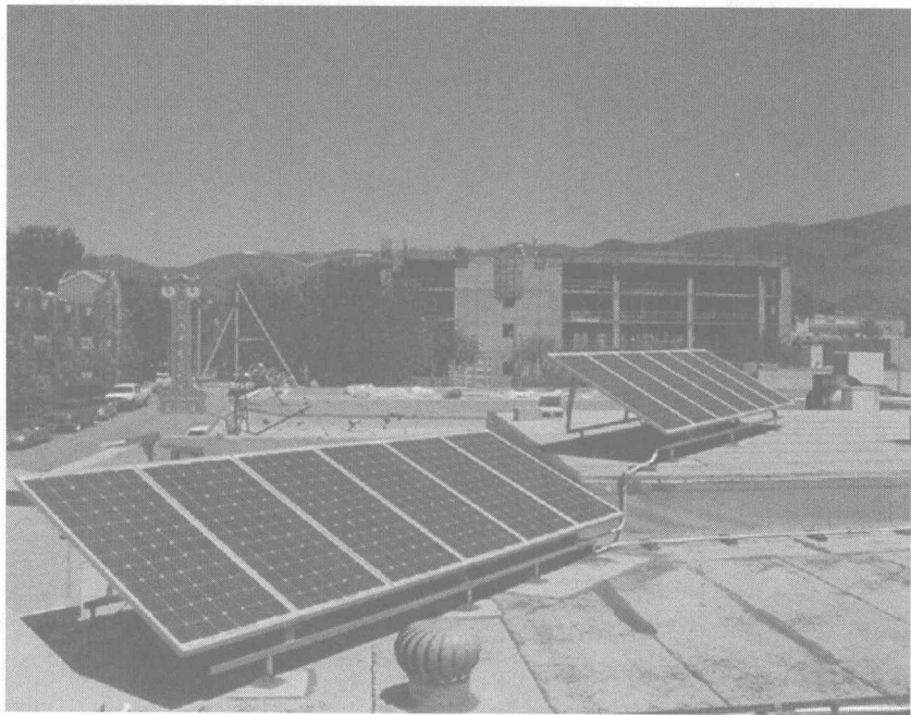
太阳能应用
